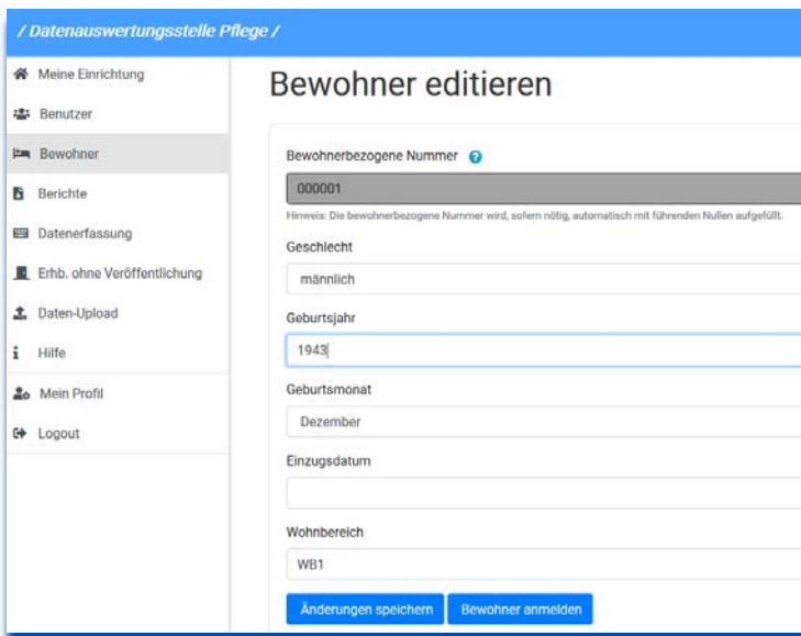
Abbildung 5: Bewohner editieren
